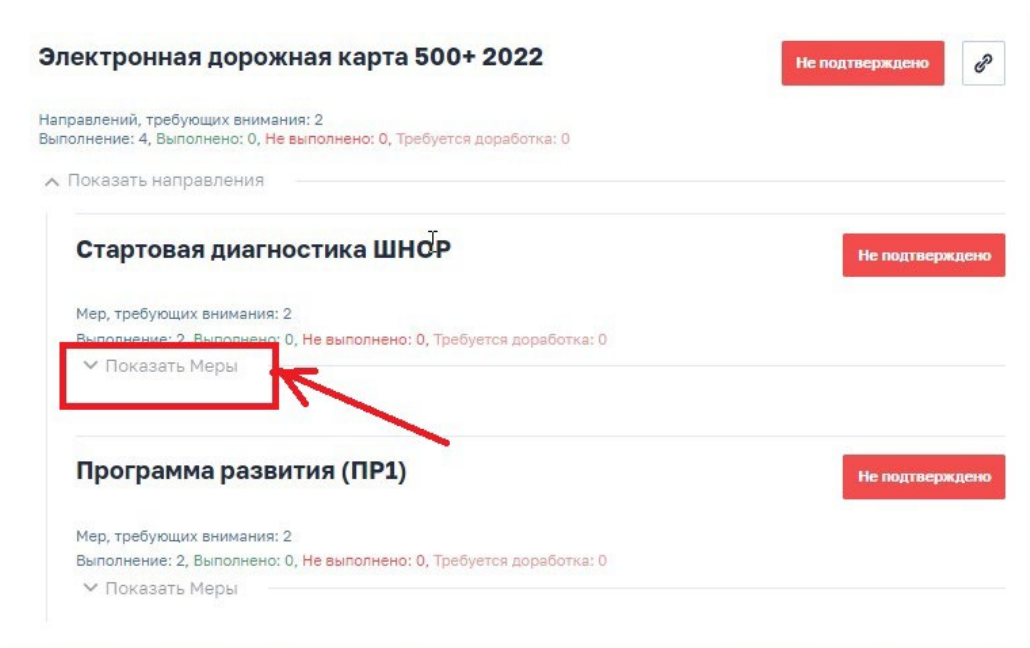
Рис. 4. Меню направления
