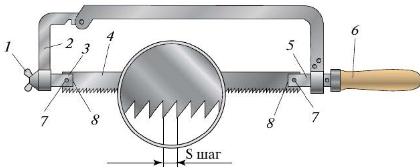
Рис. 5.24. Ручная слесарная ножовка с раздвижной рамкой
