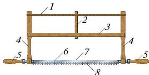
Рис. 4.2. Лучковая пила: 1 — шнур; 2 — закрутка; 3 — распорка; 4 — шаховка; 5 — ручка; 6 — полотно пилы; 7 — обушок; 8 — зубья
