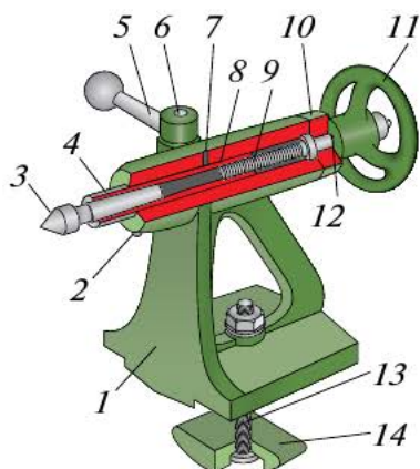
Рис. 4.9. Задняя бабка: 1 — корпус; 2 — фиксатор; 3 — центр; 4 — пиноль; 5 — рукоятка; 6 — зажим; 7 — отверстие; 8 — резьбовая втулка; 9 — винт подачи; 10 — упорная втулка; 11 — маховик; 12 — шпонка; 13 — крепёжный винт; 14 — прижимная планка
