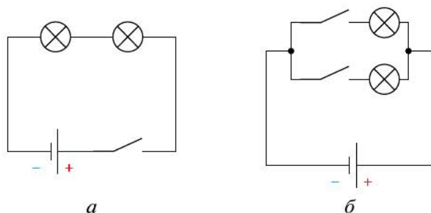
Рис. 10.12. Последовательное (а) и параллельное (б) включение ламп
