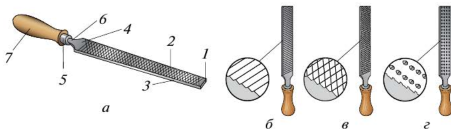
Рис. 5.32. Напильники: а — основные части: 1 — нос; 2 — ребро; 3 — грань; 4 — пятка; 5 — кольцо; 6 — хвостовик; 7 — ручка; б — одинарная (простая) насечка; в — двойная (перекрёстная) насечка; г — рапильная насечка
