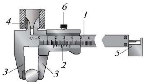
Рис. 5.12. Устройство штангенциркуля: 1 — штанга с миллиметровыми делениями; 2 — подвижная рамка с делениями (нониус); 3 — губки для измерения наружных размеров; 4 — губки для измерения внутренних размеров; 5 — глубиномер; 6 — фиксатор (фиксирующий винт)
