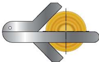
Рис. 4.19. Угловой центроискатель
