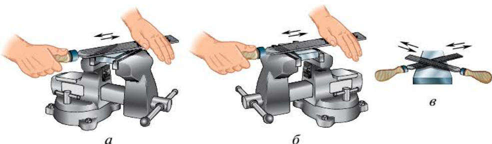
Рис. 5.40. Опиливание широких поверхностей: а — продольным штрихом; б — поперечным штрихом; в — перекрёстным штрихом
