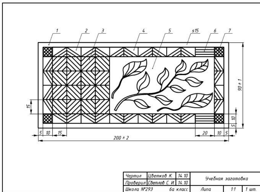
Рис. 8.7. Чертёж учебной заготовки: 1 — контурное поле; 2 — орнаментальная полоса; 3 — резное поле из 16 квадратов 15 \times 15 мм; 4 — свободные места на орнаментальной полосе; 5 — резное поле; 6 — прямоугольник; 7 — квадрат 10 \times 10 мм
