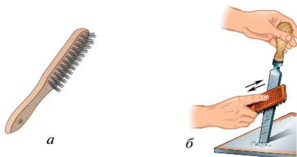
Рис. 5.39. Очистка напильника от стружки: а — корд-щётка; б — приёмы очистки
