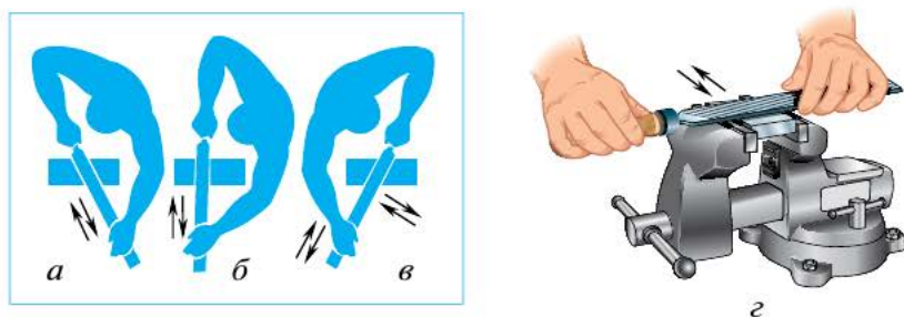
Рис. 5.37. Приёмы опиливания: а — косым штрихом; б — поперечным штрихом; в — перекрёстным штрихом; г — продольным штрихом
