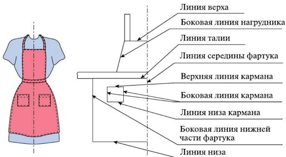
Рис. 6.29. Конструктивные линии и срезы на чертеже фартука
