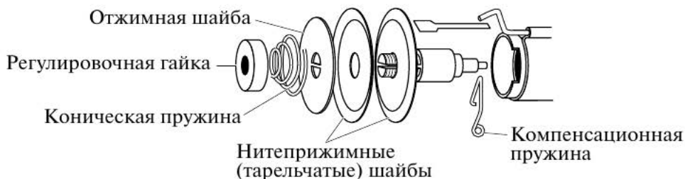
Рис. 6.16. Устройство регулятора натяжения верхней нити
