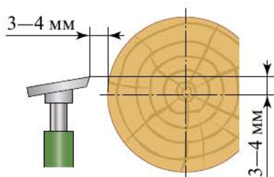
Рис. 4.33. Установка подручника
