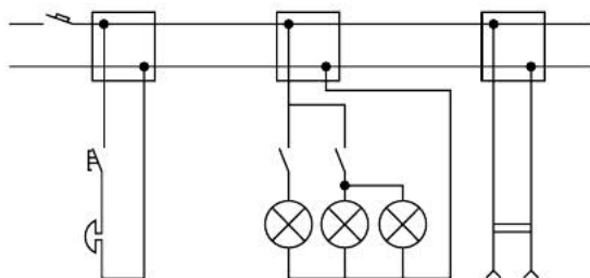
Рис. 10.13. Электрическая схема квартирной электропроводки
