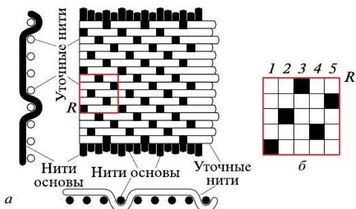
Рис. 6.10. Атласное переплетение уточное (сатин)
