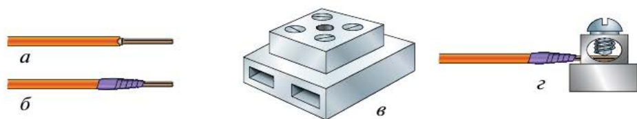
Рис. 10.2. Оконцевание многожильного провода тычком и крепление в контактном зажиме: а — зачистка провода; б — изолирование провода; в — контактный зажим; г — крепление провода
