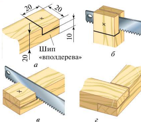
Рис. 4.59. Последовательность изготовления шипа «вполдерева»: а — разметка шипа; б — запиливание шипа; в — спливание «щёчки»; г — шип в сборе
