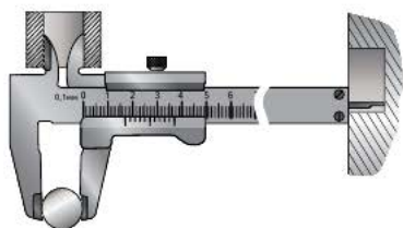
Рис. 4.16. Приёмы измерения штангенциркулем
