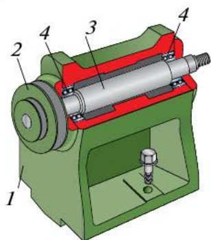
Рис. 4.8. Передняя бабка: 1 — корпус; 2 — двухступенчатый шкив; 3 — шпиндель; 4 — подшипники
