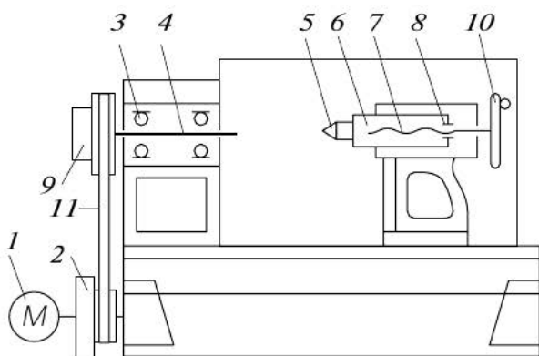
Рис. 3.6. Кинематическая схема токарного станка СТД-120М:
