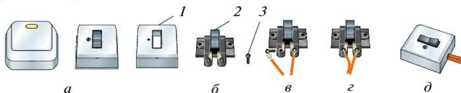
Рис. 10.7. Выключатели, их устройство и подключение: а — одно-полюсные выключатели; б — основные части выключателя (1 — крышка; 2 — основание; 3 — крепёжный винт); в — подключение одного провода, оконцованного колечком, к основанию; г — подключение двух проводов к основанию выключателя; д — выключатель в собранном виде
