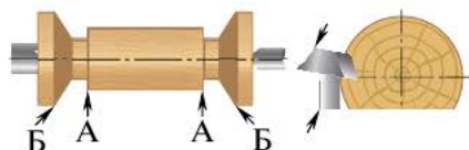
Рис. 4.39. Приёмы торцевания заготовки
