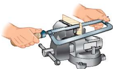
Рис. 5.30. Резание металла с поворотом ножовочного полотна
