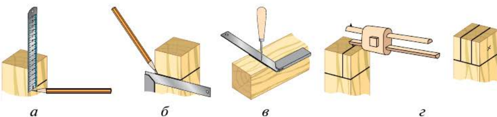
Рис. 4.52. Приёмы разметки шиповых соединений: а — линейкой и карандашом; б — угольником и карандашом; в — угольником и шилом; г — рейсмусом
