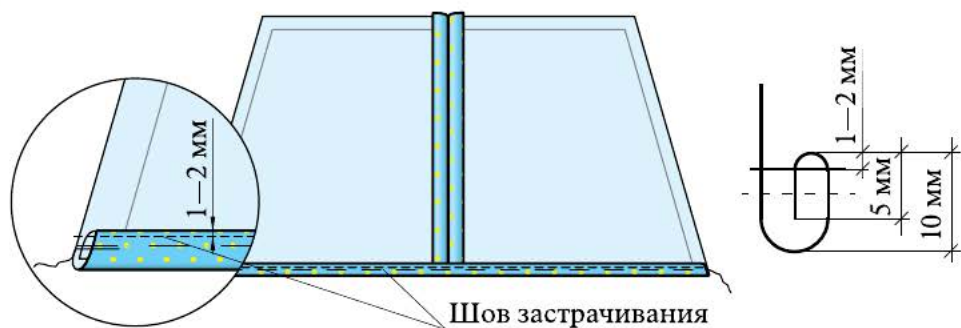
Рис. 6.48. Обработка нижнего среза обтачки
