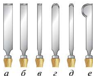
Рис. 4.26. Резцы-стамески: а, б, в — плоские; г, д — скруглённые; е — стамеска-крючок
