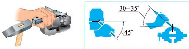
Рис. 5.20. Рубка в тисках по уровню губок
