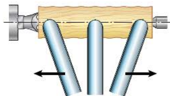
Рис. 4.34. Приёмы точения средней частью лезвия стамески
