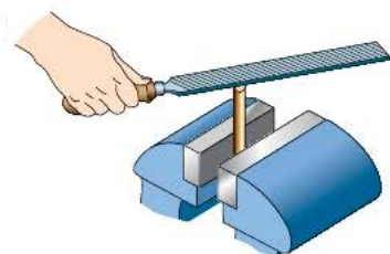
Рис. 5.58. Подготовка рабочей части паяльника
