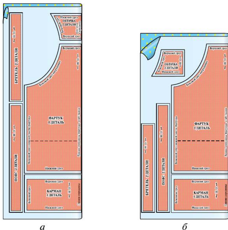
Рис. 6.42. Раскладка выкройки фартука на ткани: а — при ширине ткани 80—90 см и более; б — при ширине ткани 140—150 см
