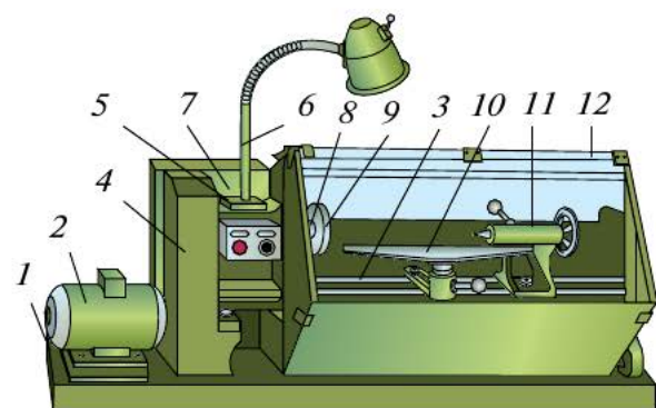
Рис. 4.7. Токарный станок для обработки древесины СТД-120М: 1 — основание; 2 — электродвигатель; 3 — станина; 4 — ограждение ремённой передачи; 5 — кнопочная станция; 6 — светильник; 7 — передняя бабка; 8 — шпиндель; 9 — планшайба; 10 — подручник; 11 — задняя бабка; 12 — защитный экран
