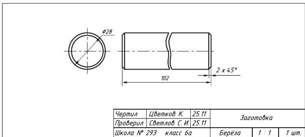
Рис. 4.41. Чертёж цилиндрической заготовки
