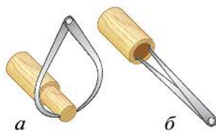
Рис. 4.17. Приёмы измерения: а — наружного размера — кронциркулем; б — внутреннего размера — нутромером
