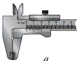
Рис. 5.14. Измерение штангенциркулем: а — проверка исправности; б — измерение
