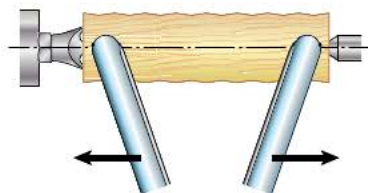
Рис. 4.35. Приёмы точения боковыми частями лезвия стамески
