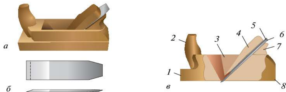
Рис. 4.4. Рубанок с деревянной колодкой: а — общий вид рубанка; б — железка (нож); в — основные части рубанка: 1 — колодка; 2 — передняя ручка-рожок; 3 — леток; 4 — деревянный клин; 5 — стружколом; 6 — нож; 7 — упор; 8 — подошва
