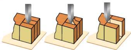
Рис. 4.58. Последовательность долбления сквозной проушины
