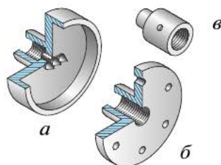
Рис. 4.28. Крепёжные приспособления: а — трезубец; б — планшайба; в — патрон-стакан
