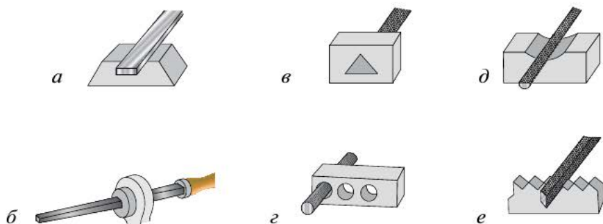
Рис. 5.33. Профили напильников: а — плоский; б — квадратный; в — треугольный; г — круглый; д — полукруглый; е — ромбический
