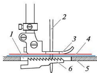
Рис. 6.19. Взаимодействие прижимной лапки и зубчатой рейки:
