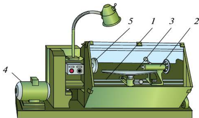
Рис. 4.11. Токарный станок для обработки древесины
