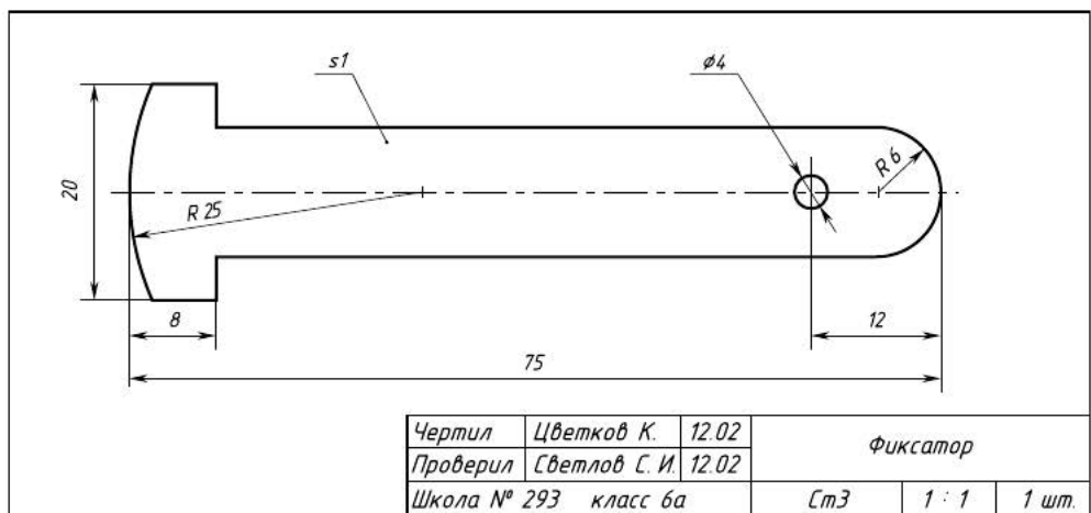
Рис. 5.41. Чертёж фиксатора
