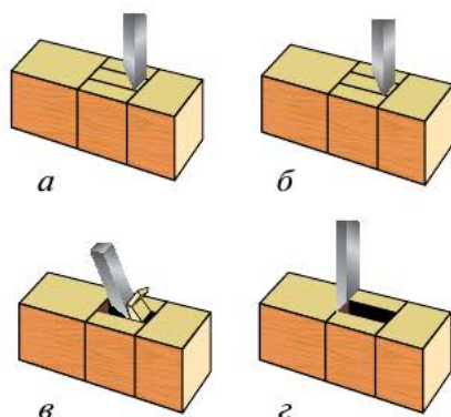
Рис. 4.57. Последовательность долбления гнезда
