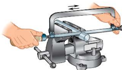
Рис. 5.29. Резание ножовкой прутка круглого сечения
