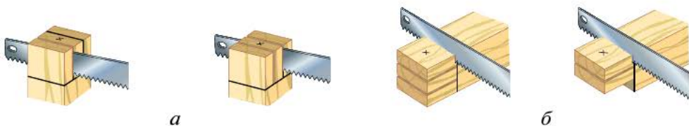
Рис. 4.53. Приёмы запиливания проушин и шипов: а — запиливание проушины; б — запиливание шипов (удаление «щёчек»)
