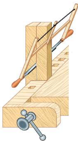
Рис. 4.3. Приём пиления лучковой пилой вдоль волокон
