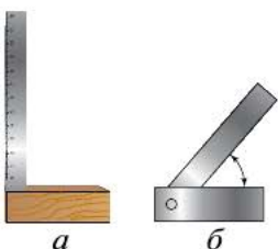
Рис. 4.18. Инструменты для угловых измерений: а — угольник; б — ярунок
