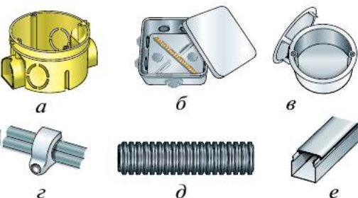
Рис. 10.10. Виды установочных изделий: а — коробка установочная; б — коробка ответвления; в — распаячная коробка; г — скоба для провода; д — труба гофрированная; е — короб пластмассовый (кабель-канал)
