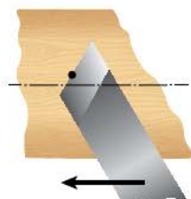
Рис. 4.36. Приём точения стамеской с косым срезом
