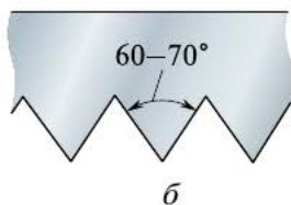
Рис. 3.23. Форма зубьев пил для пиления: а — продольного; б — поперёк и вдоль волокон; в — смешанного
