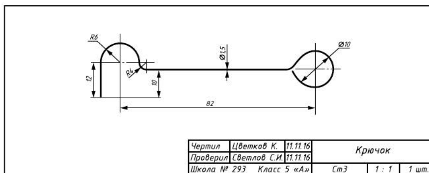
Рис. 4.12. Чертёж крючка
