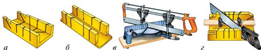
Рис. 3.25. Приспособления для точного пиления заготовок из древесины: а — стусло П-образное; б — стусло Ч-образное; в — стусло поворотное; г — приём пиления заготовки под углом 45°
