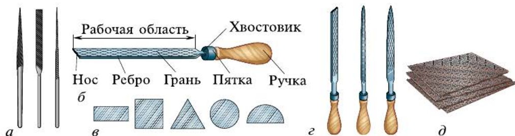
Рис. 3.26. Инструменты для зачистки, чистовой обработки и шлифовки заготовок из древесины: а — надфили; б — основные части напильника; в — формы сечения напильников; г — рашпили; д — шлифовальная шкурка
