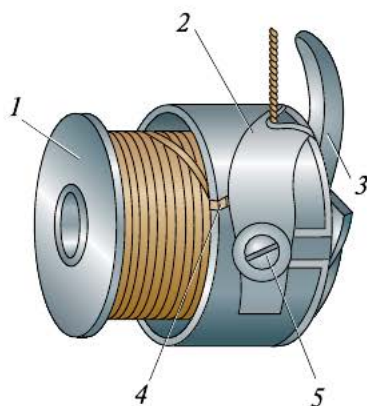
Рис. 5.23. Устройство шпульного колпачка: 1 — шпулька; 2 — пластинчатая пружина; 3 — установочный палец; 4 — косая прорезь; 5 — регулировочный винт
