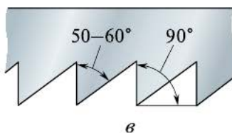
Рис. 3.23. Форма зубьев пил для пиления: а — продольного; б — поперёк и вдоль волокон; в — смешанного
