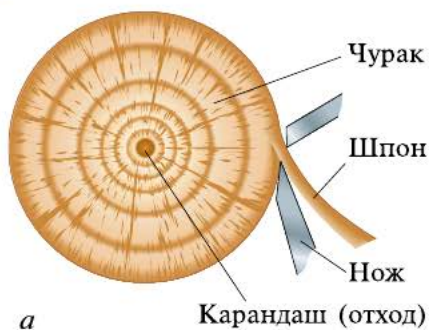
Рис. 3.12. Шпон: а — схема получения лущёного шпона; б — изделие, декорированное различными видами шпона
