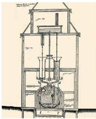
Рис. 9.11. Чертёж и модель машины И. И. Ползунова
