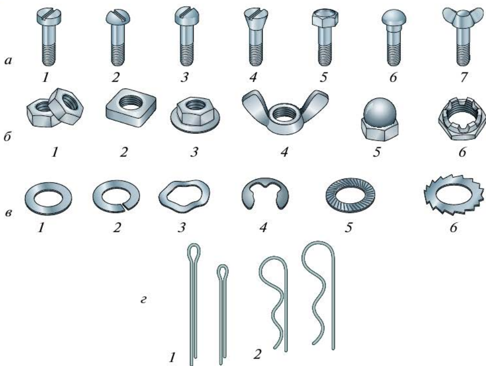
Рис. 4.40. Крепёжные детали: а — болты: 1 — с цилиндрической головкой; 2 — с полукруглой головкой; 3 — с полупотайной головкой; 4 — с потайной головкой; 5 — с шестигранной головкой; 6 — с плоско-выпуклой головкой; 7 — барашковый; б — гайки: 1 — шестигранная; 2 — квадратная; 3 — шестигранная с фланцем; 4 — барашковая; 5 — колпачковая; 6 — корончатая низкая; в — шайбы: 1 — плоская; 2 — пружинная Гровера; 3 — волновая; 4 — быстросъёмная; 5 — с насечкой; 6 — стопорная; г — шплинты: 1 — прямые; 2 — пружинные
