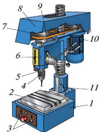
Рис. 4.33. Настольный сверлильный станок: 1 — станина; 2 — стол; 3 — кнопки пуска и остановки электродвигателя; 4 — патрон; 5 — шпиндель; 6 — шпиндельная бабка; 7 — шкив ступенчатый; 8 — защитный кожух; 9 — ремень приводной; 10 — электродвигатель; 11 — штурвал ручной подачи шпинделя
