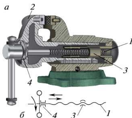
Рис. 2.3. Винтовые механизмы в слесарных тисках: а — внешний вид; б — изображение на кинематической схеме; 1 — винт; 2 — подвижная губка; 3 — гайка; 4 — подшипник скольжения
