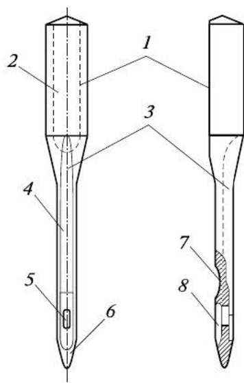
Рис. 5.19. Машинная игла:
