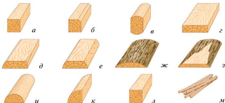
Рис. 3.10. Основные виды пиломатериалов: а — четырёхкантный брус; б — четырёхкантный брус с обзолом; в — двухкантный брус; г — обрезная доска; д — полуобрезная доска; е — необрезная доска; ж — горбыльный обзол; з — дощатый обзол; и — пластина; к — четвертина; л — брусок; м — рейки
