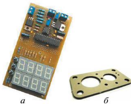
Рис. 4.32. Изделия из листового текстолита: а — печатная плата; б — прокладка карбюратора
