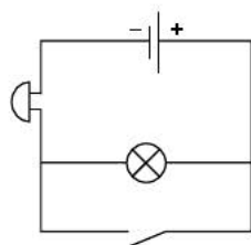
Рис. 10.37. Электрическая схема логической операции НЕ
