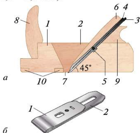
Рис. 3.29. Рубанок с двойной железкой: а — общий вид: 1 — колодка; 2 — леток; 3 — нож; 4 — стружколом; 5 — винт крепления стружколома; 6 — клин; 7 — роток; 8 — рожек; 9 — упор; 10 — вставки из твёрдой древесины; б — железка в собранном виде: 1 — контржелезка; 2 — железка (нож)
