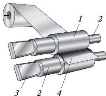
Рис. 4.21. Валки прокатные листовые:
