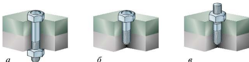
Рис. 4.39. Резьбовые соединения: а — болтовое; б — винтовое; в — соединение шпилькой
