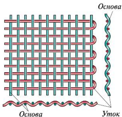
Рис. 5.6. Полотняное переплетение
