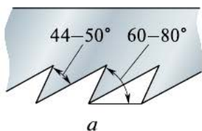
Рис. 3.23. Форма зубьев пил для пиления: а — продольного; б — поперёк и вдоль волокон; в — смешанного
