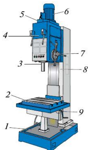
Рис. 4.34. Вертикально-сверлильный станок напольного типа: 1 — плита; 2 — стол; 3 — шпиндель; 4 — коробка подач; 5 — защитный кожух; 6 — электродвигатель; 7 — штурвал ручной подачи шпинделя; 8 — станина; 9 — рукоятка вертикального перемещения стола
