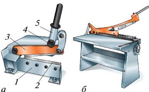
Рис. 4.26. Рычажные ножницы: а — настольные: 1 — корпус; 2 — нож неподвижный; 3 — нож подвижный; 4 — ось; 5 — рычаг; б — напольные
