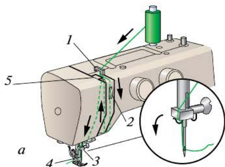
Рис. 5.25. Последовательность заправки верхней нити: 1 — верхний нитенаправитель; 2 — регулятор натяжения верхней нити; 3 — нижний нитенаправитель; 4 — игла; 5 — рычаг нитепритягивателя
