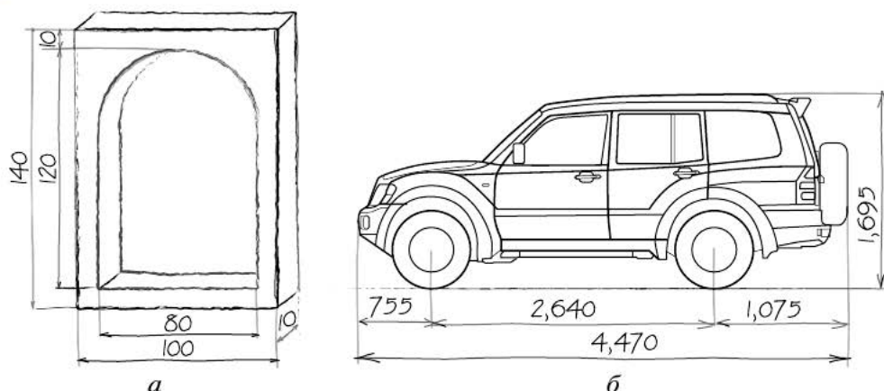
Рис. 1.15. Технические рисунки: а — рамки для фотографий; б — автомобиля
