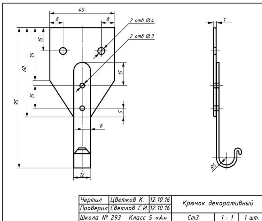
Рис. 4.43. Сборочный чертёж декоративного крючка
