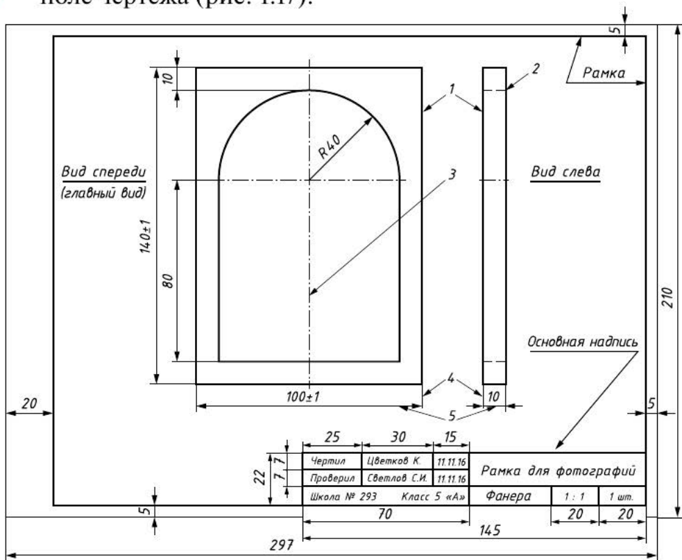
Рис. 1.17. Оформление чертежа: 1 — сплошная основная толстая (линия видимого контура); 2 — штриховая (линия невидимого контура); 3 — штрихпунктирная тонкая (осевая); 4 — сплошная тонкая (выносная); 5 — сплошная тонкая (размерная)
