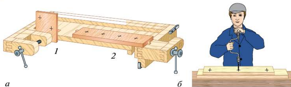
Рис. 3.37. Сверление: а — крепление заготовок при сверлении: 1 — в переднем зажиме верстака; 2 — в заднем зажиме верстака; б — рабочая поза при сверлении коловоротом
