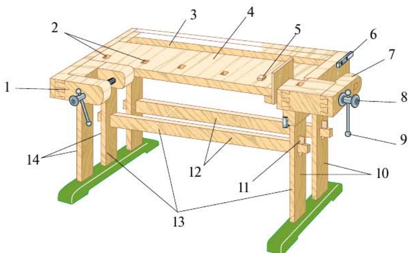
Рис. 3.1. Основные части столярного верстака:
