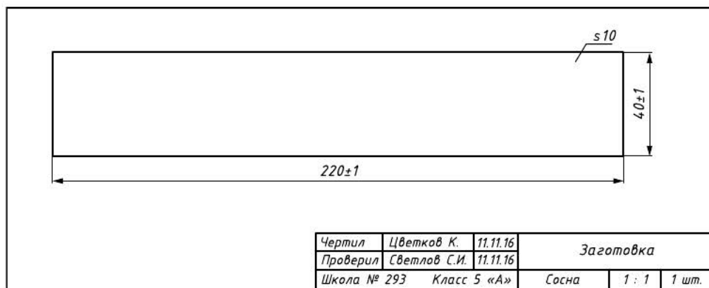
Рис. 3.34. Чертёж заготовки хозяйственной лопаточки
