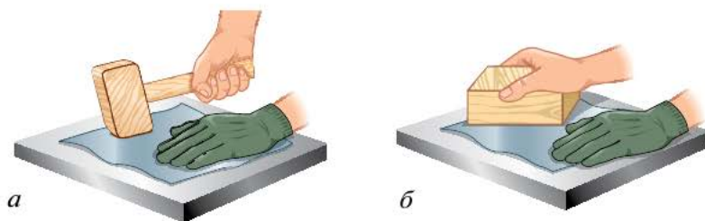
Рис. 4.28. Правка заготовки из тонколистового металла на плите: а — киянкой; б — бруском
