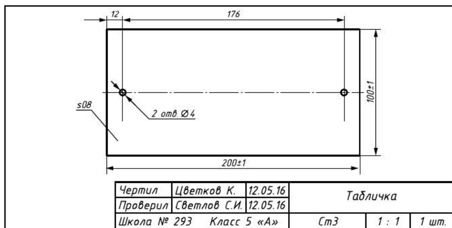
Рис. 4.31. Чертёж металлической таблички
