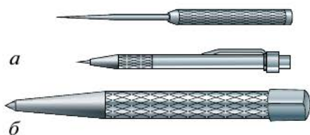
Рис. 4.6. Инструменты для разметки: а — чертилки; б — кернер
