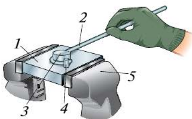
Рис. 4.16. Гибка проволоки в приспособлении в слесарных тисках: 1 — приспособление; 2 — заготовка; 3 — оправка; 4 — упор; 5 — слесарные тиски
