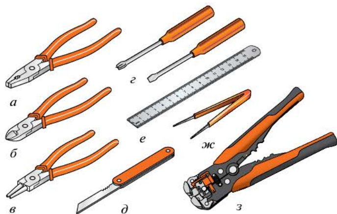
Рис. 10.14. Электромонтажные инструменты: а — пассатижи; б — бокорезы; в — круглогубцы; г — отвёртки; д — нож; е — линейка металлическая; жс — пинцет монтажный; з — приспособление для снятия изоляции с проводов
