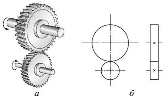
Рис. 2.4. Цилиндрическая зубчатая передача: а — наглядное изображение; б — изображение на кинематической схеме
