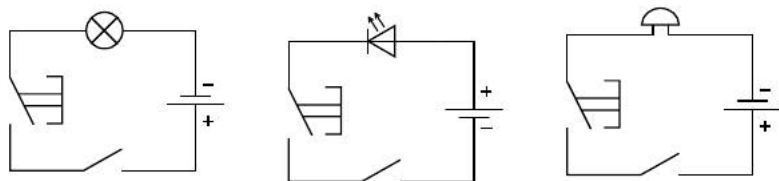
Рис. 10.35. Электрические схемы логической операции И
