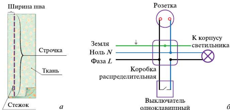
Рис. 1.16. Типы схем: а — схема машинного шва; б — схема соединения розетки, выключателя и светильника
