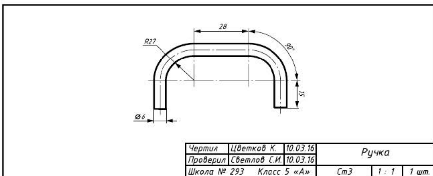
Рис. 4.13. Чертёж ручки
