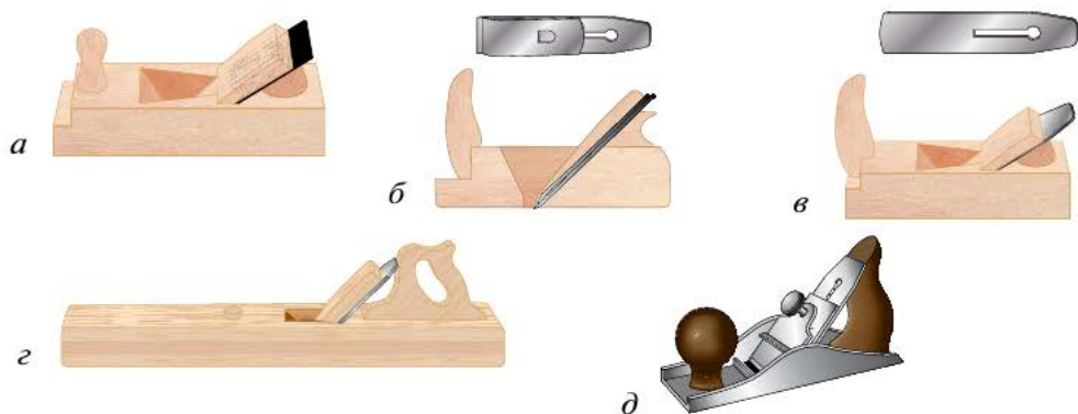
Рис. 3.28. Инструменты для строгания древесины: а — рубанок с одинарной железкой; б — рубанок с двойной железкой; в — шерхебель; г — фуганок; д — рубанок металлический
