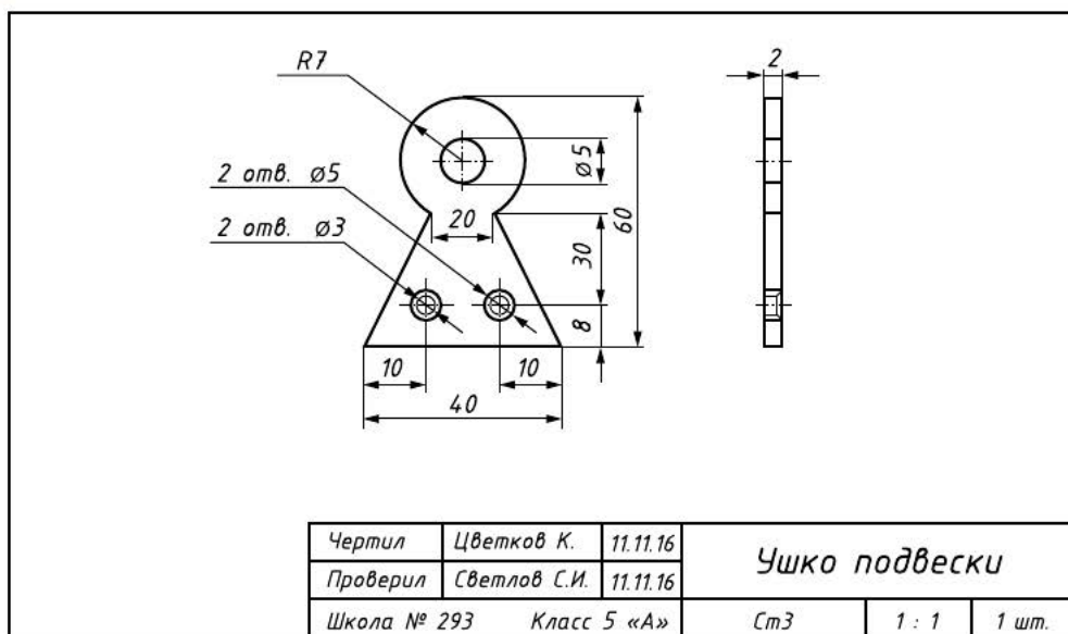
Рис. 1.11. Чертёж однодетального изделия
