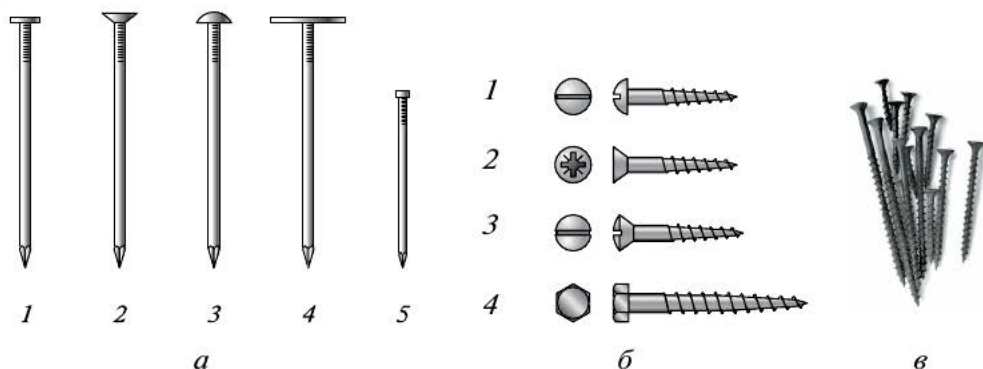
Рис. 3.39. Крепёжные изделия для соединения деталей из древесины: а — гвозди с головками разной формы: 1 — с плоской головкой; 2 — с потайной головкой; 3 — с полупотайной головкой; 4 — кровельный; 5 — отделочный; б — шурупы: 1 — полукруглый; 2 — потайной; 3 — полупотайной; 4 — шестигранный; в — саморезы по дереву
