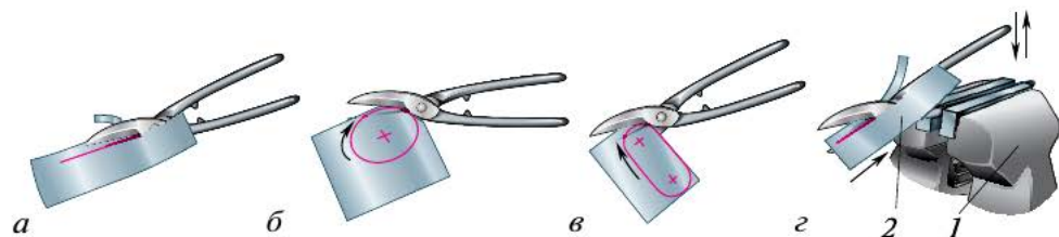
Рис. 4.30. Приёмы резания слесарными ножницами: a — резание заготовки на весу по прямой линии; б, в — вырезание заготовок сложных форм; г — резание заготовки в слесарных тисках
