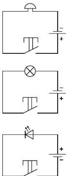
Рис. 10.25. Электрические схемы модели аппарата Морзе
