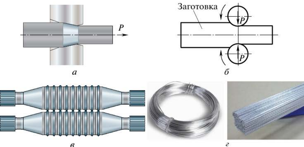
Рис. 4.9. Производство проволоки: а — волочение; б — прокатка; в — валки прокатного стана; г — транспортировка проволоки в мотках и прутках
