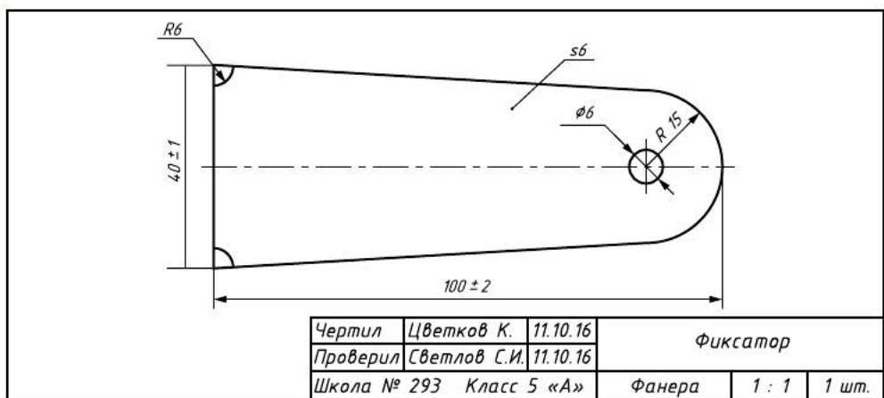
Рис. 7. Чертёж фиксатора
