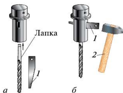
Рис. 4.36. Приёмы установки и удаления сверла с коническим хвостовиком: а — крепление сверла в шпинделе станка; б — удаление сверла клином: 1 — клин; 2 — молоток
