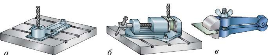
Рис. 4.37. Способы крепления заготовок: а — на столе станка с помощью прижимной пластины; б — в машинных тисках; в — в ручных слесарных тисочках
