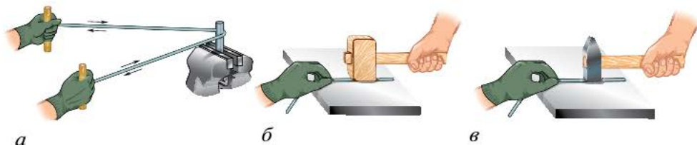
Рис. 4.11. Приёмы правки проволоки: а — на оправке; б — киянкой по плите; в — слесарным молотком по плите
