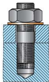
Рис. 2.6. Резьбовое соединение
