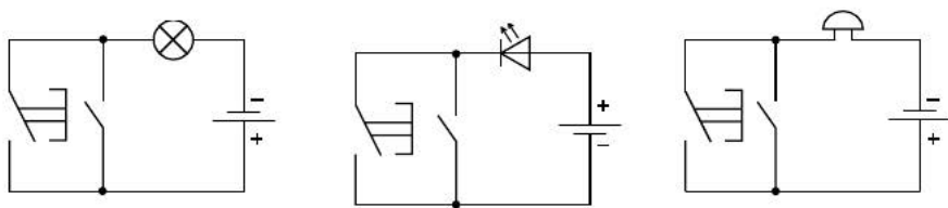
Рис. 10.36. Электрические схемы логической операции ИЛИ
