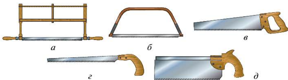
Рис. 3.21. Ручные инструменты для пиления: а — лучковая пила с деревянной рамкой; б — пила садовая лучковая; в — столярная ножовка широкая; г — пила выкружная узкая; д — ножовка обушковая прорезная
