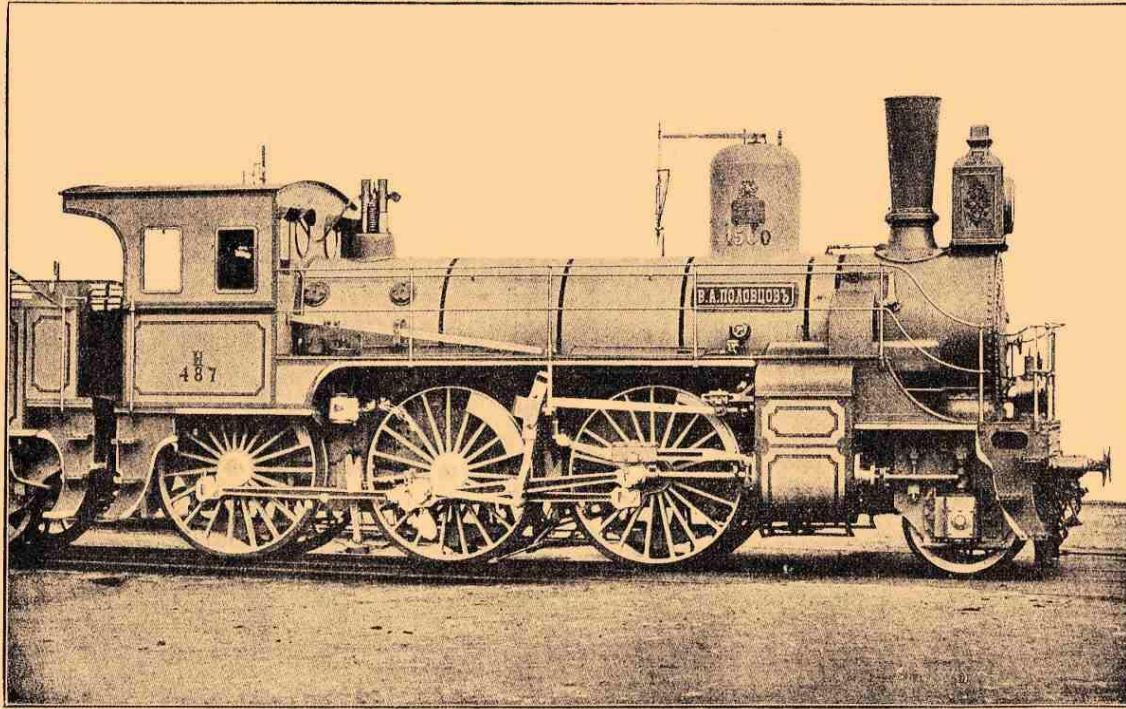
Четырехосный паровоз командь, съ одной поддерживающей осью, серия H Николаевской жел. дор.
