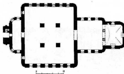
План церкви
